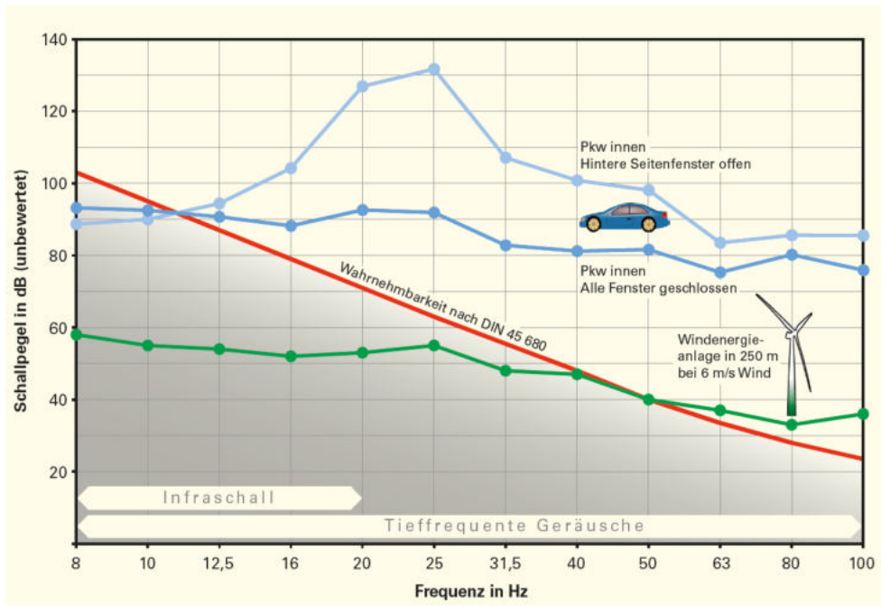
Abbildung 3: Infraschall von WEA und PKW im Vergleich (LUBW & LGA Baden-Württemberg (Darstellung) /13/ und LfU Bayern (Daten) /8/)
